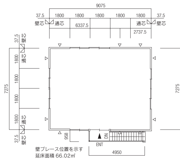
2F 平面図
