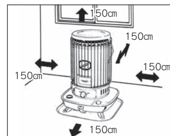
対流式ストーブ
