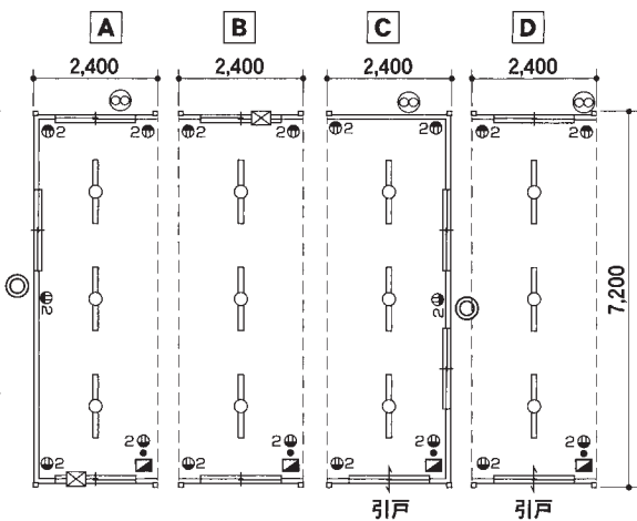
SH-HP72 平面図
