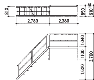
SH-HP型/階段
