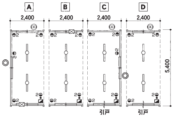
SH-HP54 平面図
