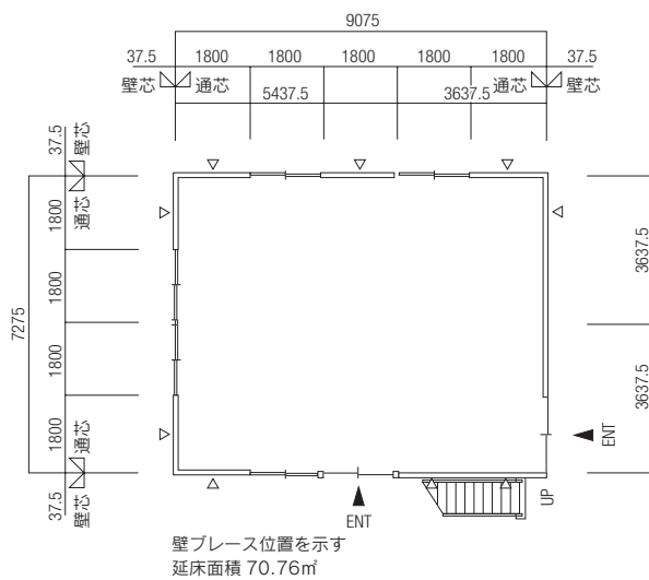
1F 平面図
