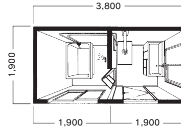
フロハウス B-1型
